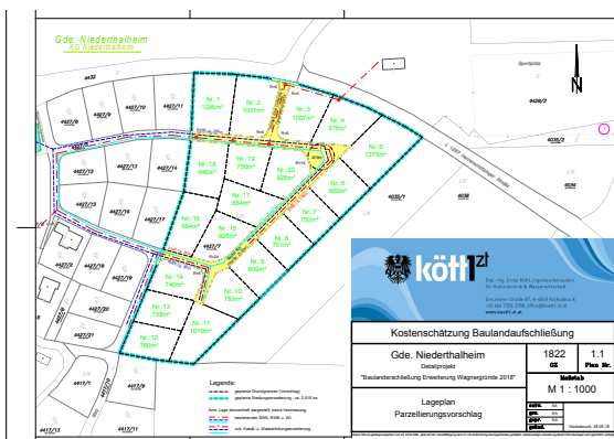
Projektstudie Erweiterung Siedlungsraum Sportplatzstraße
